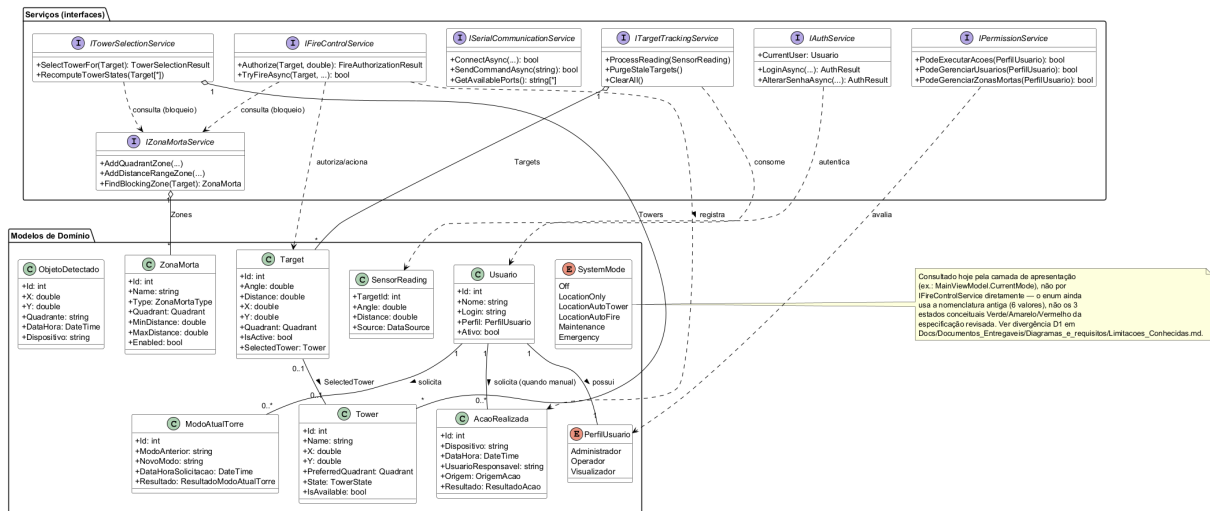
Figure 1: Diagrama de classes do RadarTorres.
