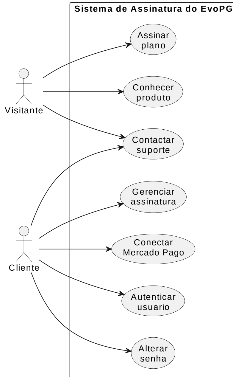
Figura 4 – Diagrama de casos de uso do site de assinatura
