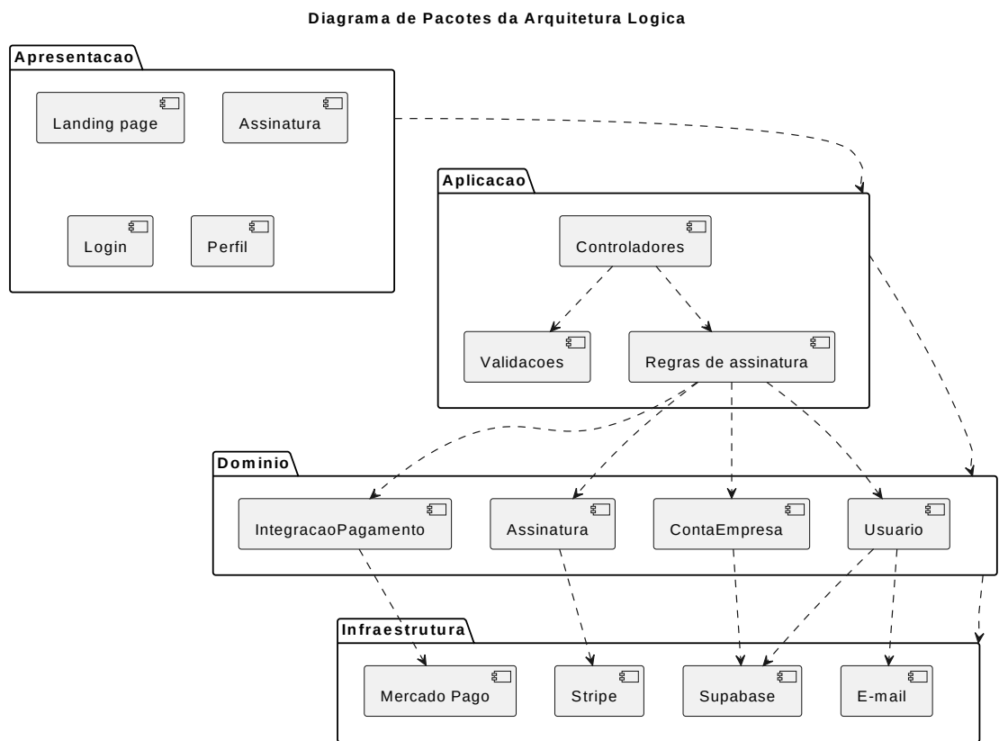
Figura 10 – Diagrama de pacotes da arquitetura lógica
