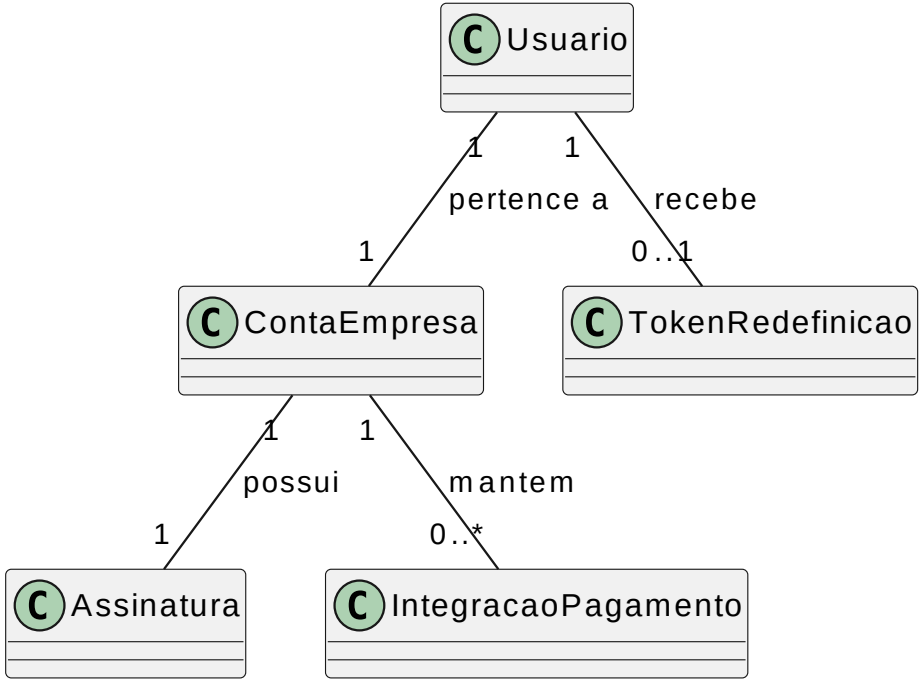
Diagrama de Classes do Domínio Principal do Site de Assinatura
