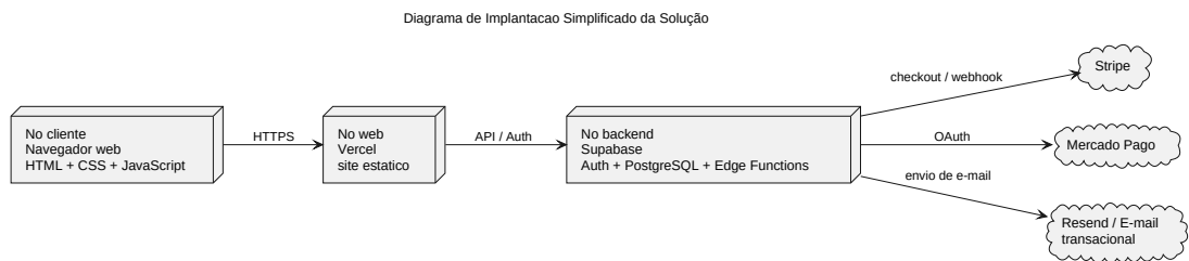
Figura 11 – Diagrama de implantação simplificado da solução
