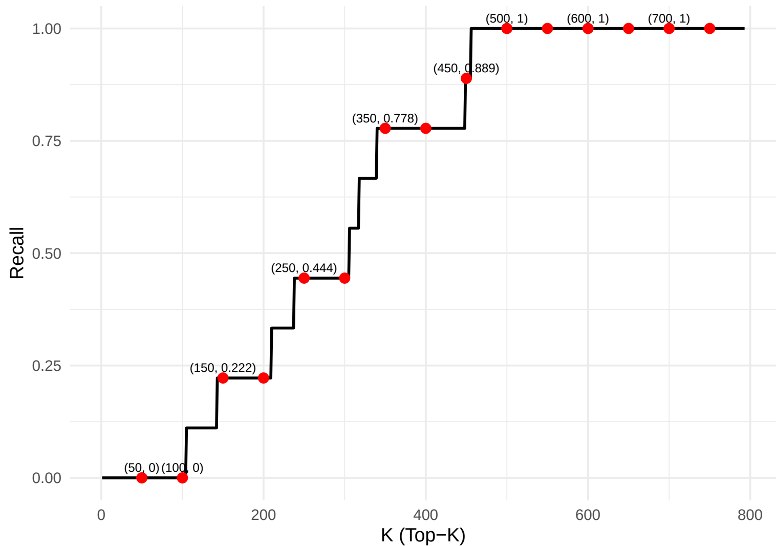
Recall@K para MDD
