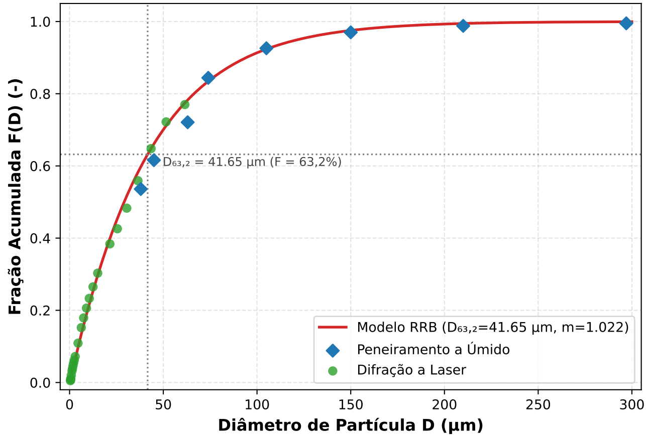
(a) Fração Mássica Acumulada Passante F(D) - Escala Linear
