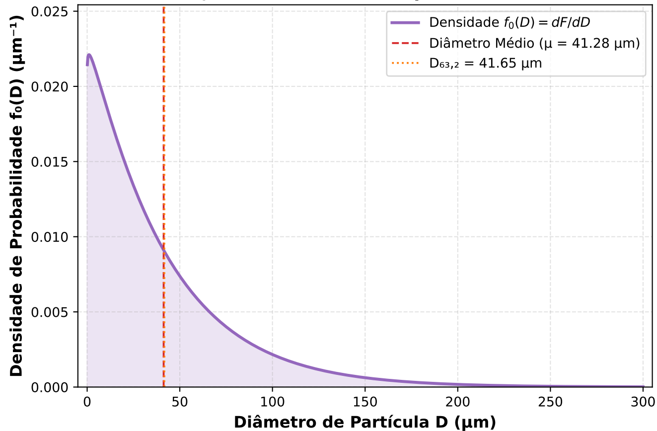
(c) Função Densidade de Frequência Inicial f_0(D)
