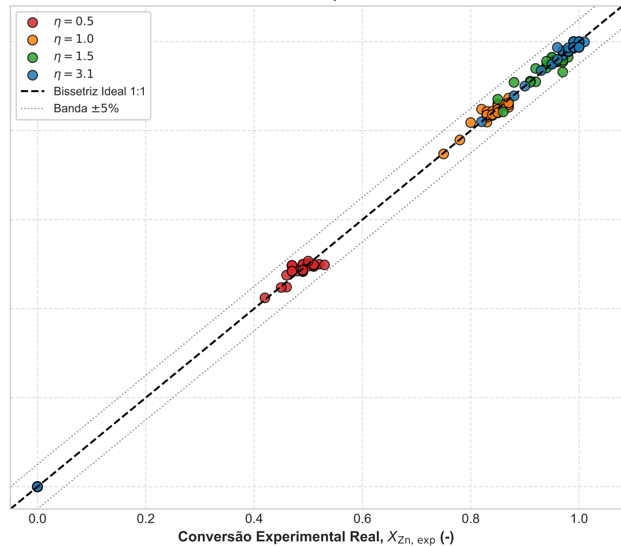
Painel (b) — Nova Abordagem Híbrida / Adaptativa
