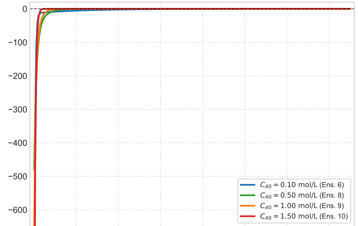
Painel (b) — Taxa de Retração v(t) para \eta = 1.0
