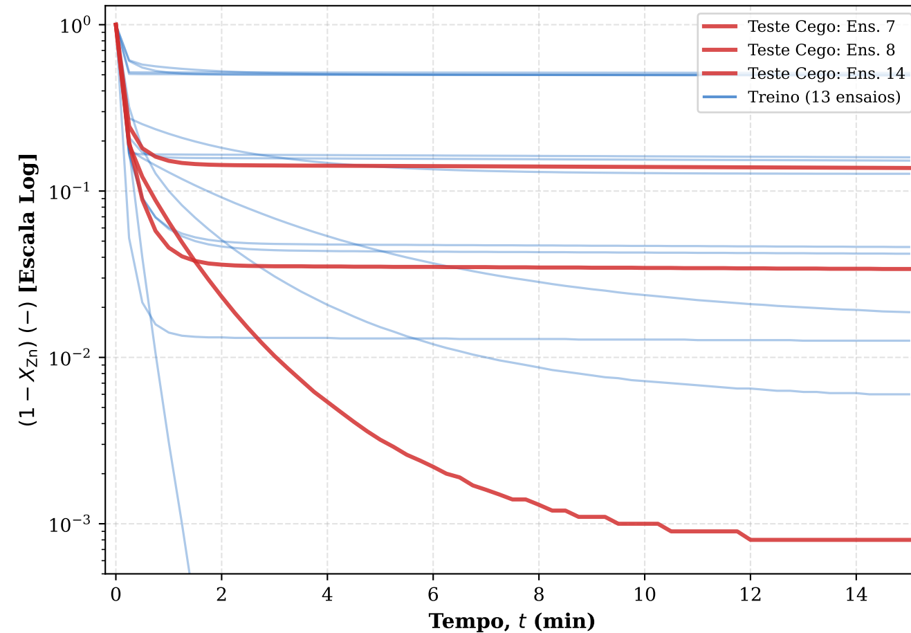
(c) Fração Residual ( 1 - X_{Zn} ) [Escala Semilogarítmica]
