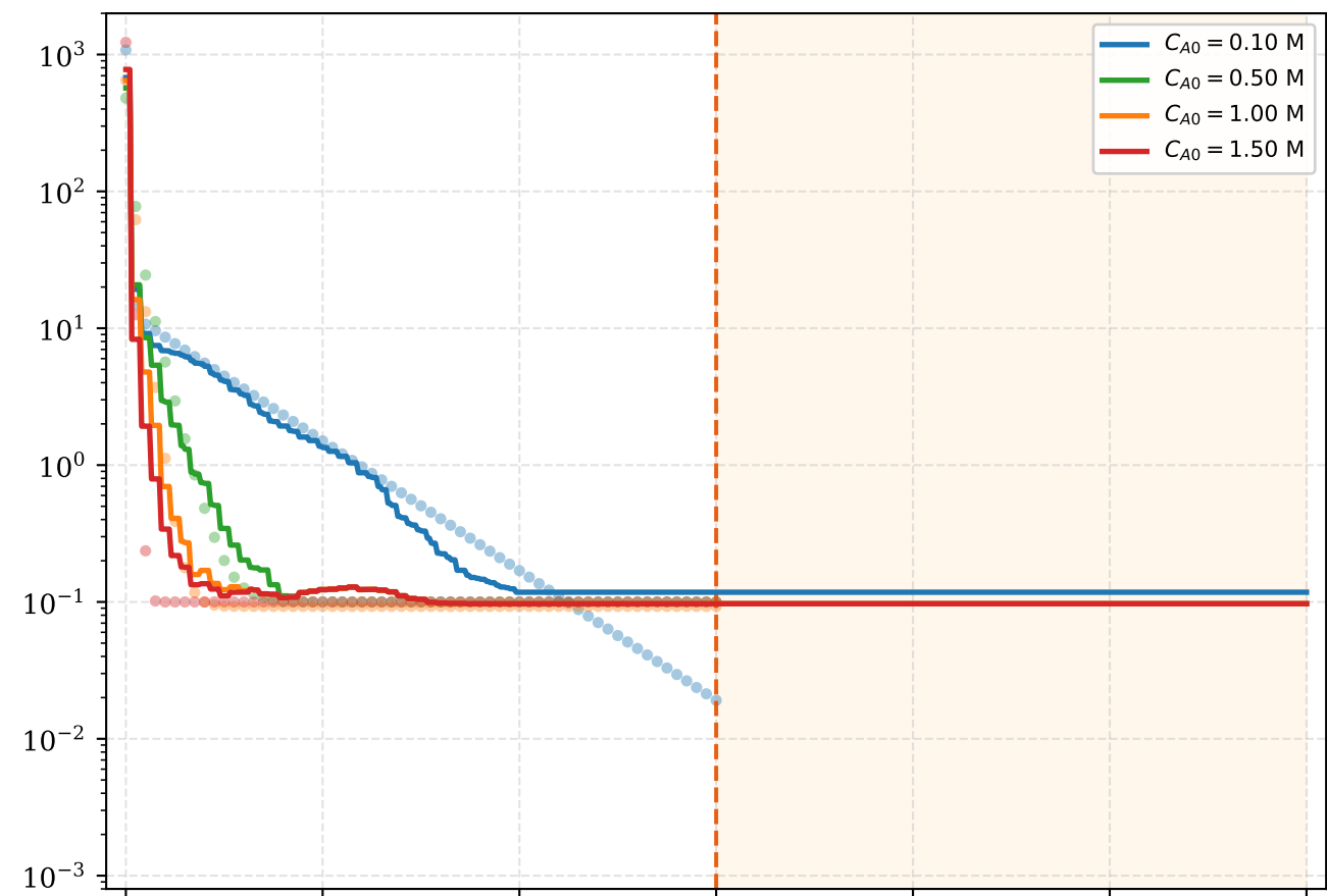
Painel (d) — Razão Molar \eta = 3.1
