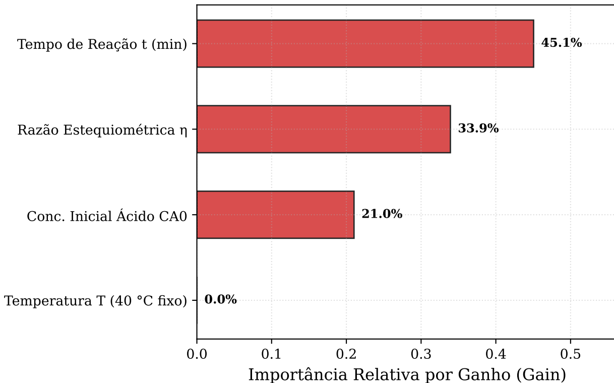
(a) Ganho Médio de Divisão (Treino)
