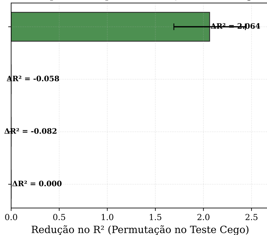
(b) Importância por Permutação (Teste Cego)
