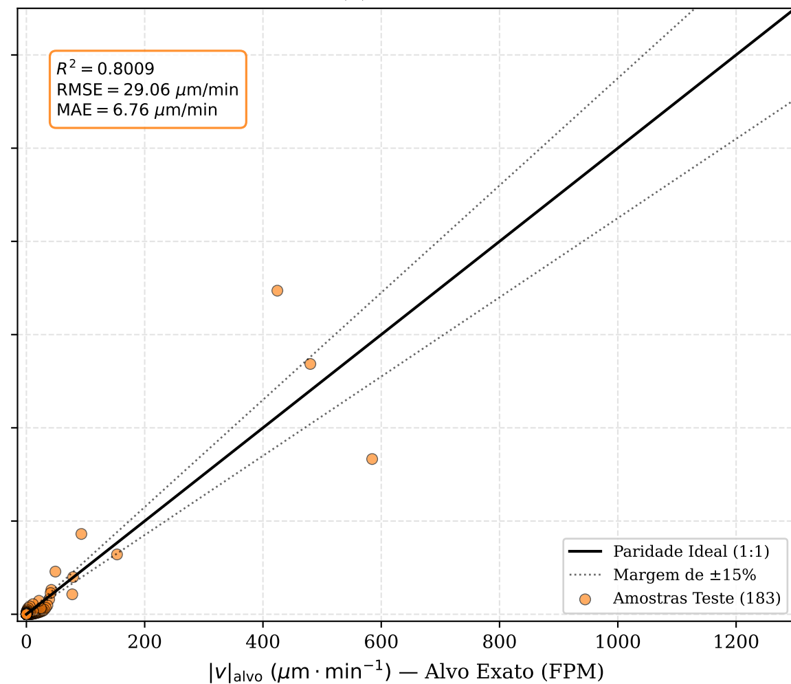
(d) XGBoost
