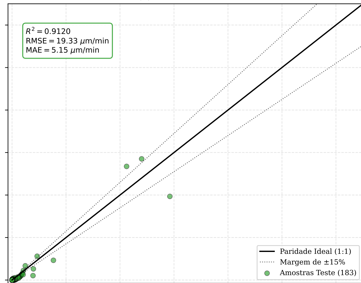
(d) XGBoost
