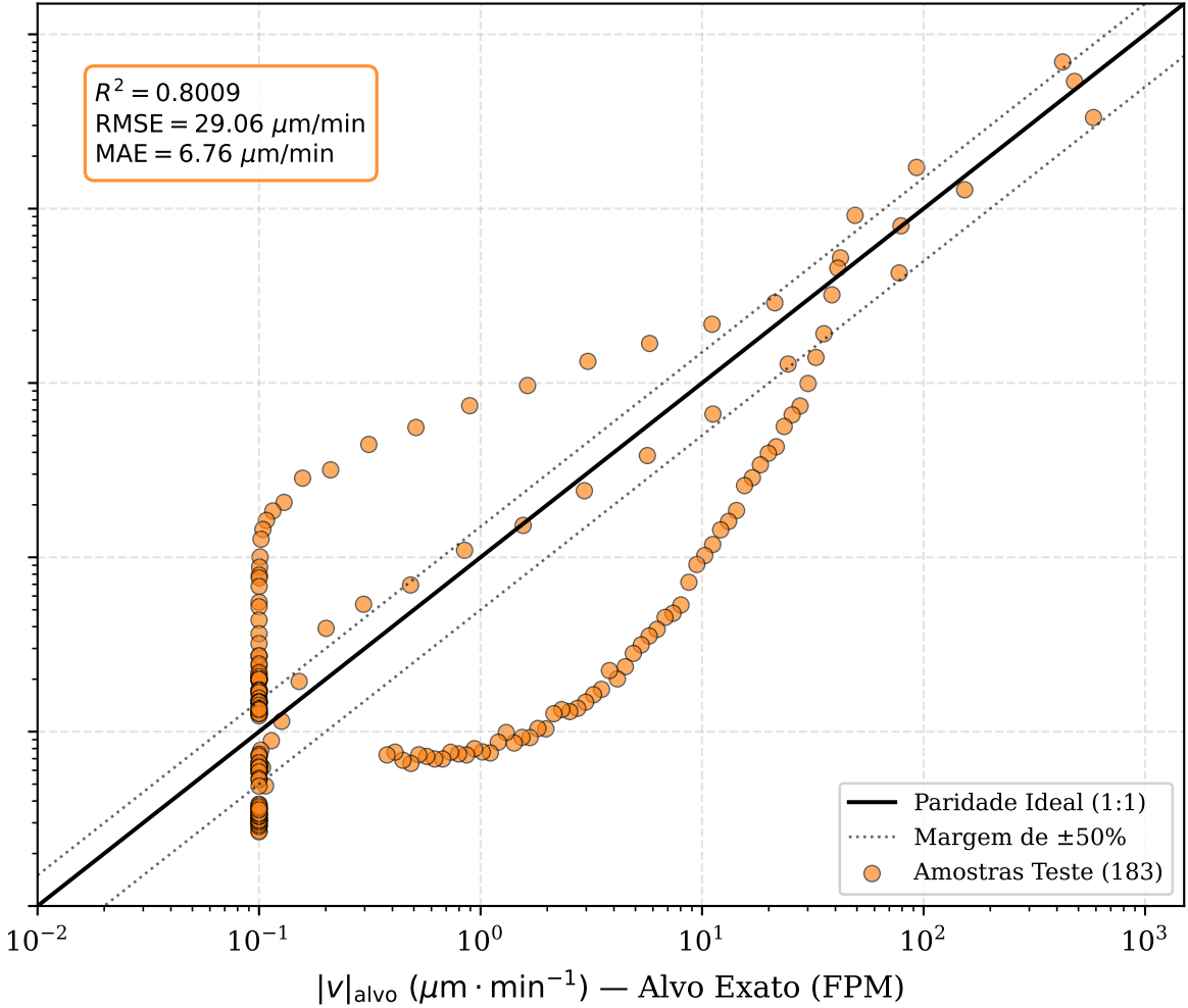
(d) XGBoost
