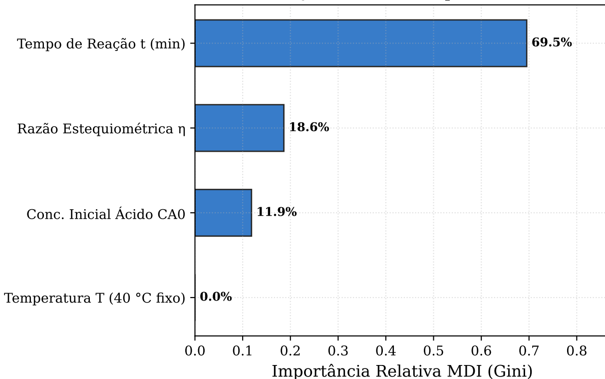
(a) Redução Média de Impureza (Treino)
