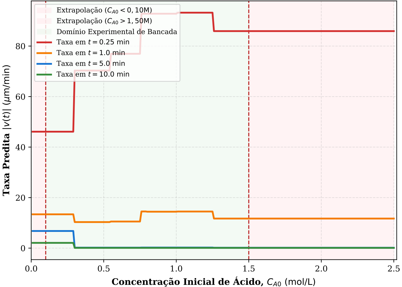
(a) Efeito da Acidez C_{A0} com \eta = 1,5 (Saturação de Borda nas Árvores)
