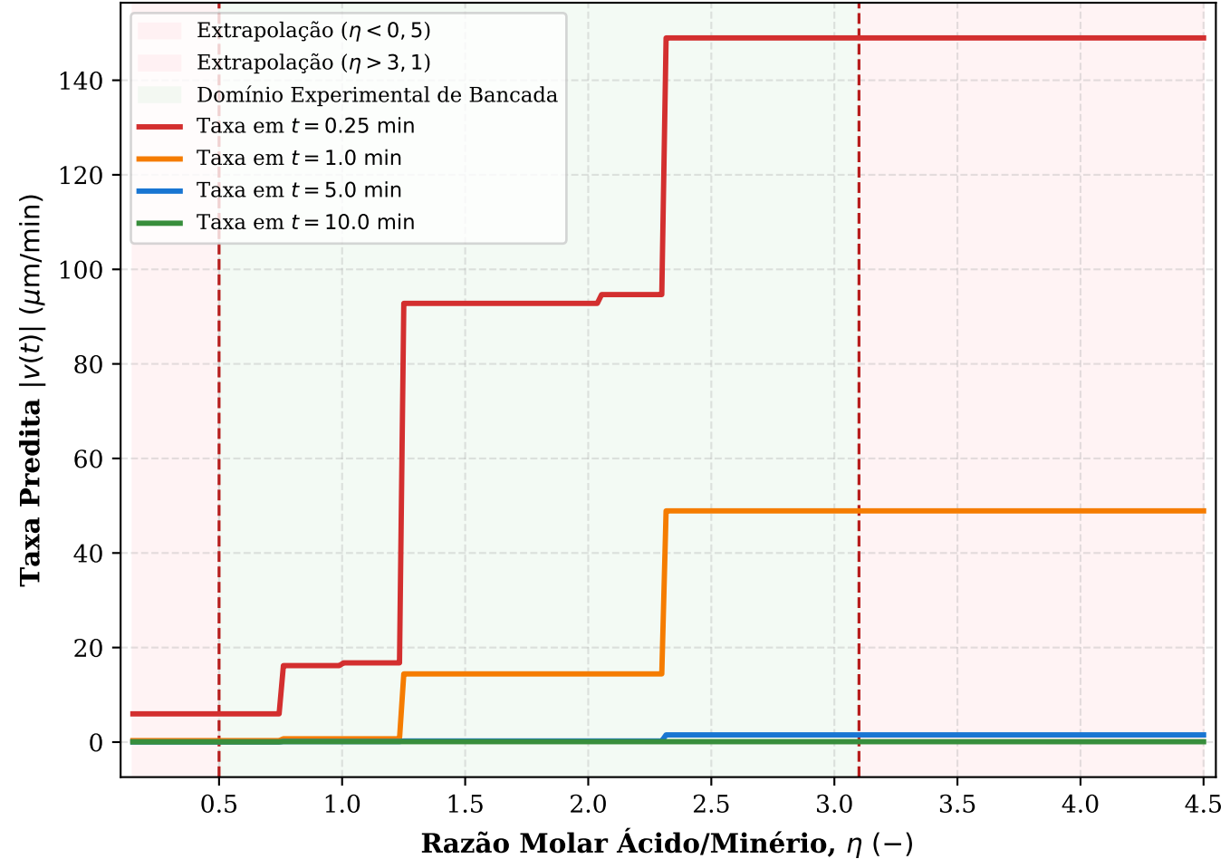
(b) Efeito da Razão Molar \eta com C_{A0} = 1,00\text{M} (Saturação de Borda nas Árvores)
