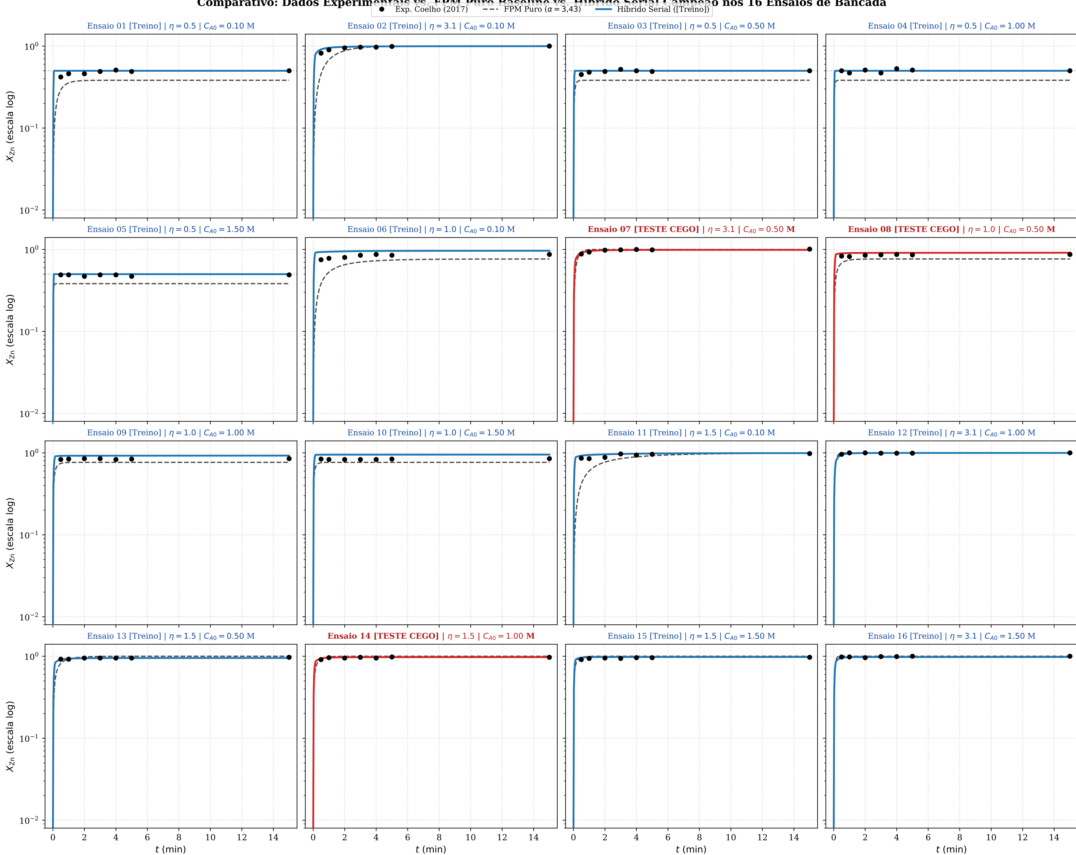
Figura 12a (Semilog X_{Zn} ): Cinética de Conversão X_{Zn}(t) em Escala Semilogarítmica Comparativo: Dados Experimentais vs. FPM Puro Baseline vs. Híbrido Serial Campeão nos 16 Ensaios de Bancada
