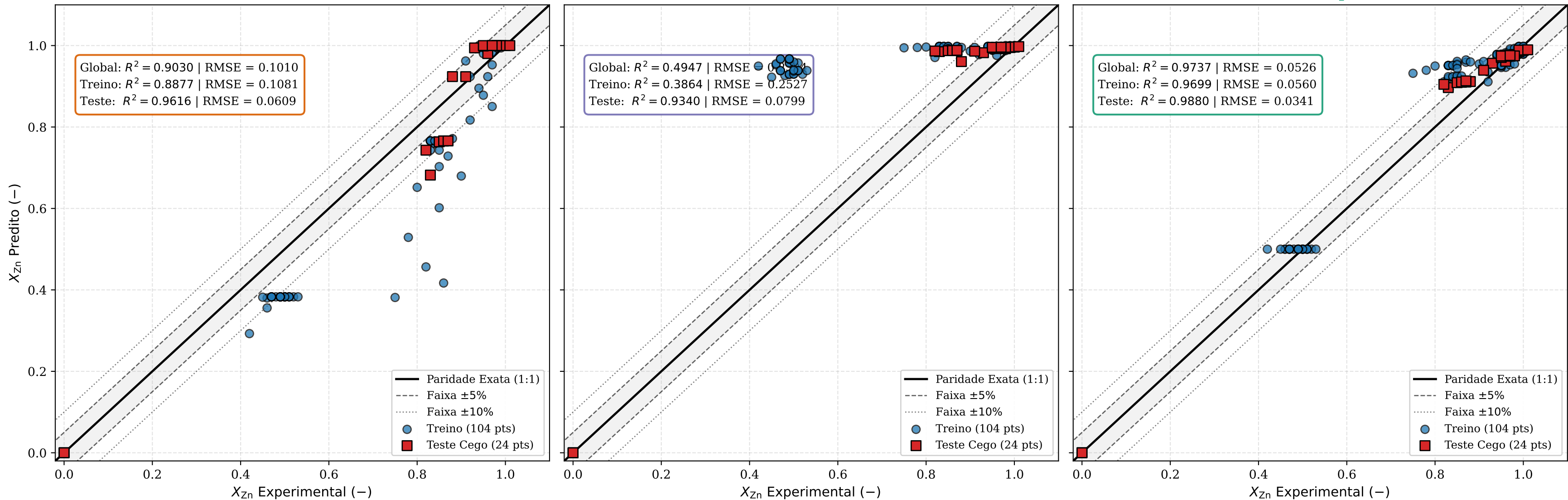
Figura 12b: Diagramas de Paridade 1:1 para a Conversão de Zinco X_{Zn} (128 Pontos Experimentais)
