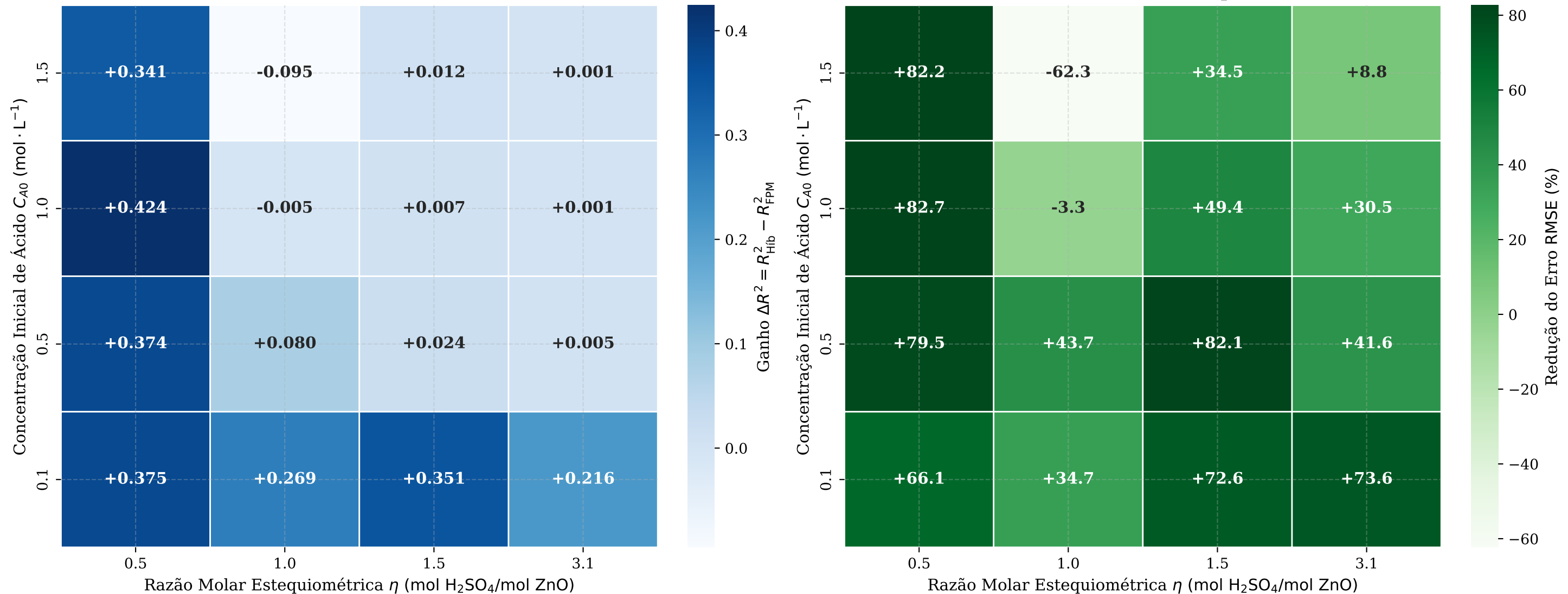
Figura 12d: Mapa Térmico do Ganho Relativo do Híbrido Serial sobre o FPM Baseline no Espaço Operacional ( C_{A0} \times \eta ) (a) Ganho em R^2 do Híbrido Serial sobre o FPM Puro (b) Redução Percentual do Erro RMSE pelo Híbrido Serial (%)
