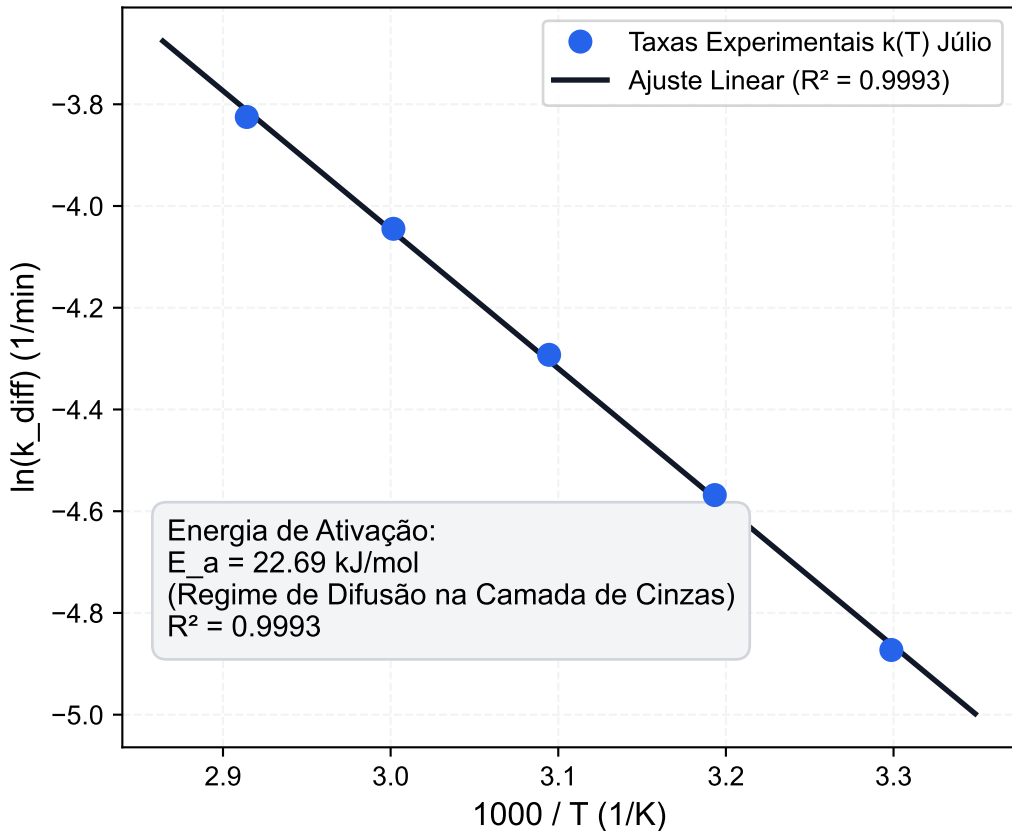
Figura 13b — Linearização de Arrhenius (Balarini 2009)
