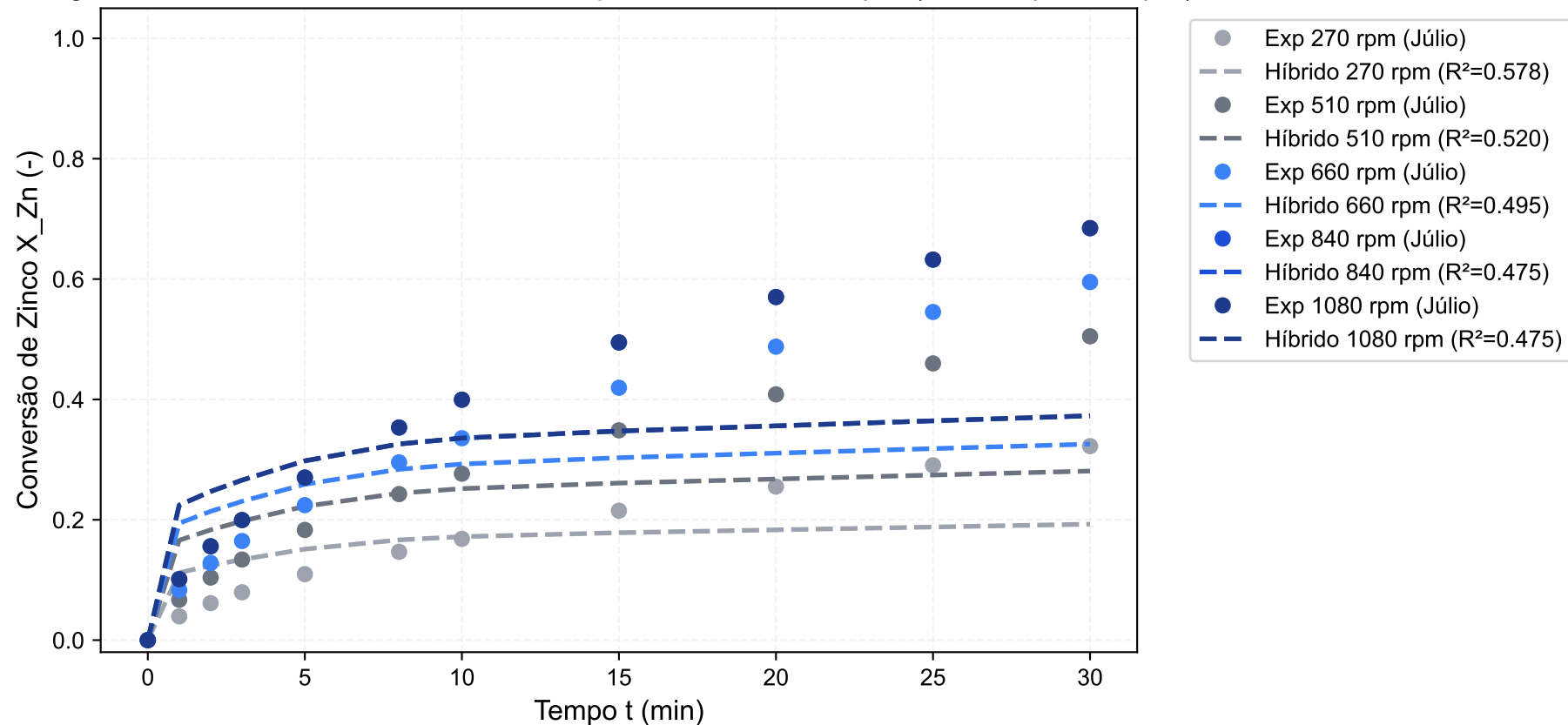
Figura 13e — Efeito Hidrodinâmico: Rotação de 270 a 1080 rpm (30 °C, dp = 180 µm)
