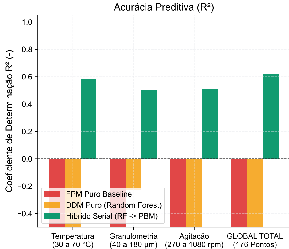
Figura 13g — Comparativo Global de Acurácia: FPM vs. DDM vs. Híbrido nos Dados de Júlio Balarini
