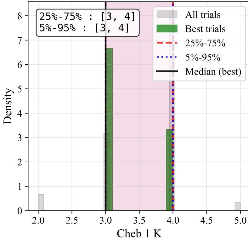
Cheb 1 K
