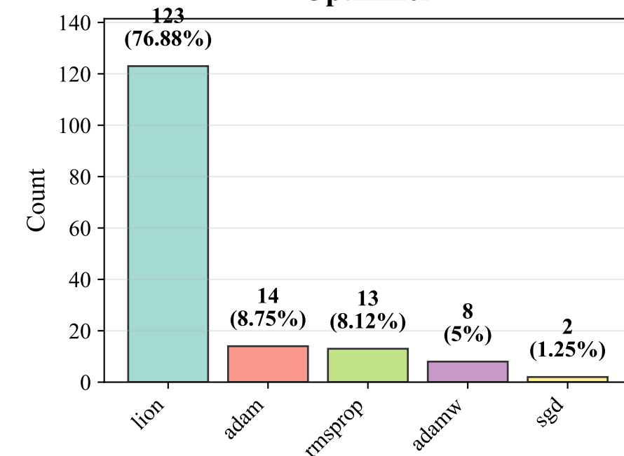
Optimizer
