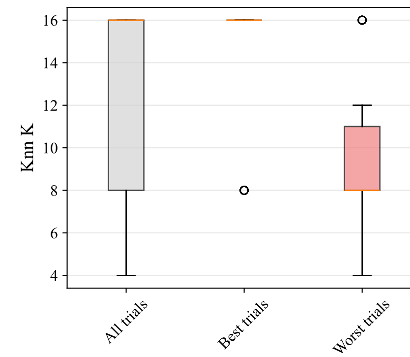
Knn K
