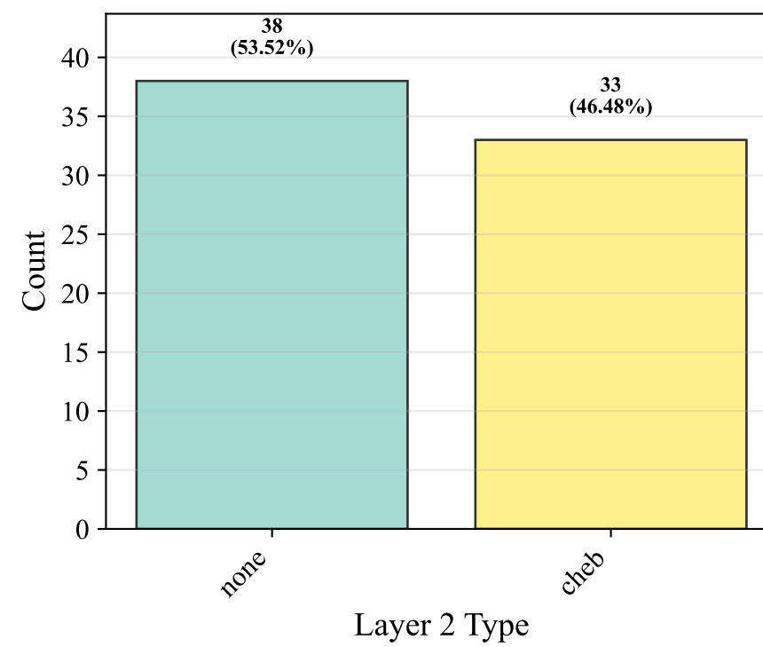
Layer 2 Type
