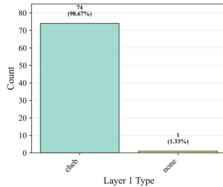
Layer 1 Type
