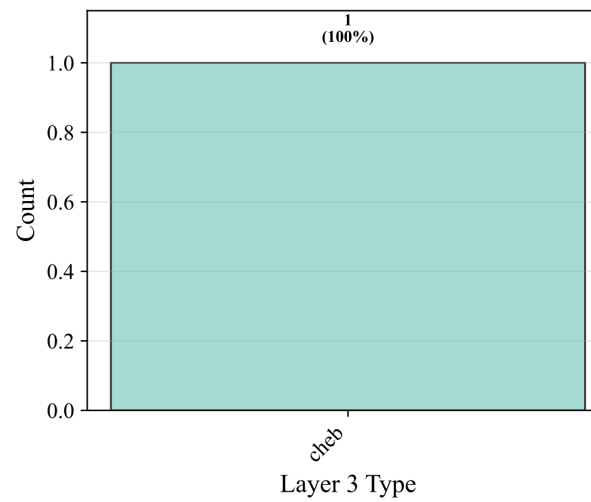
Layer 3 Type
