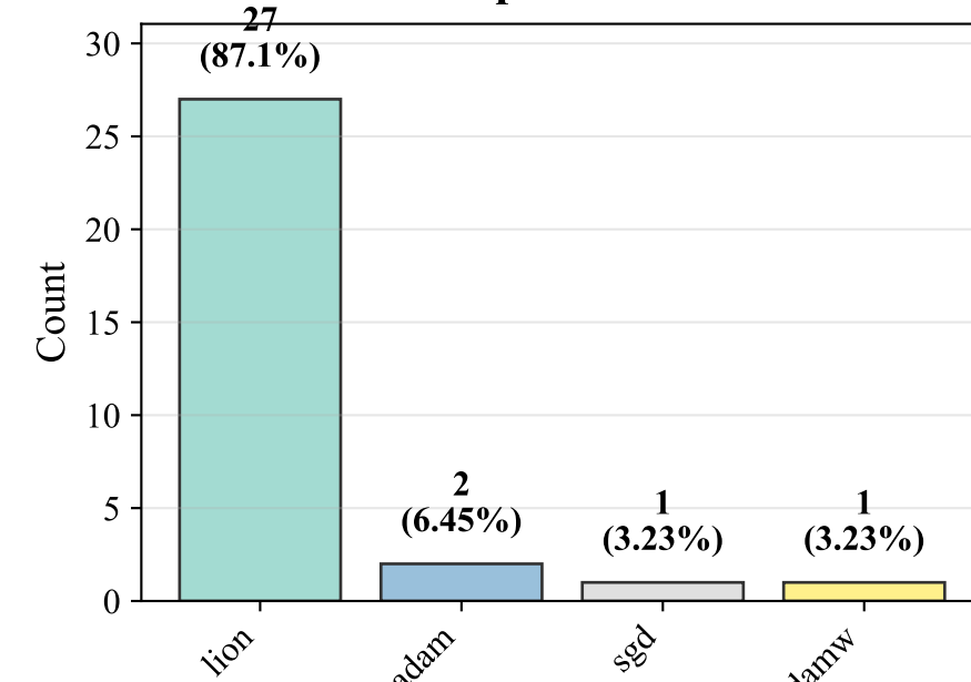
Optimizer
