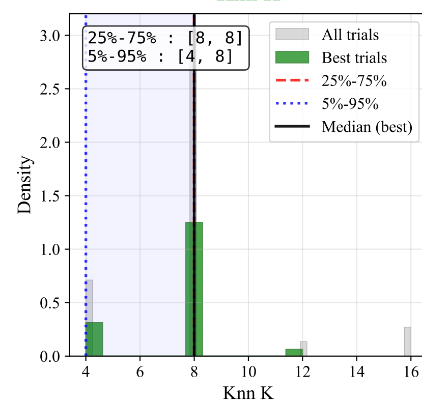
Knn K
