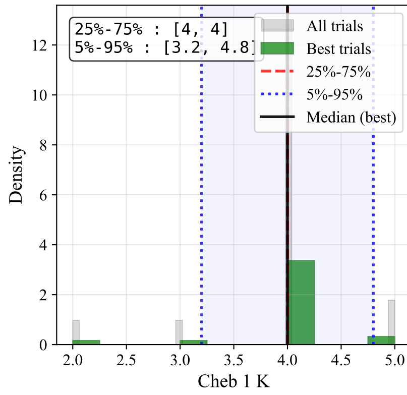
Cheb 1 K
