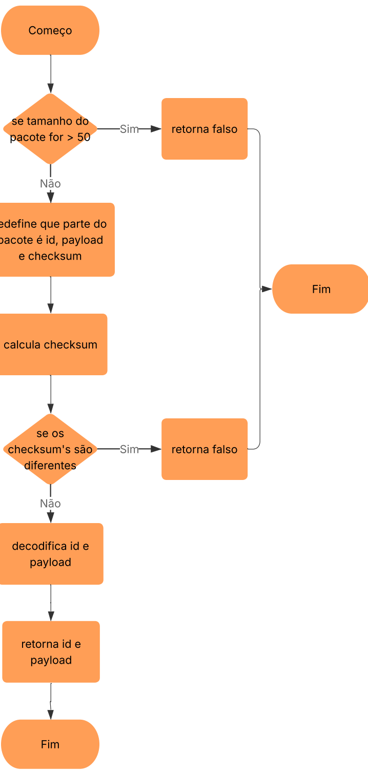
função validar
