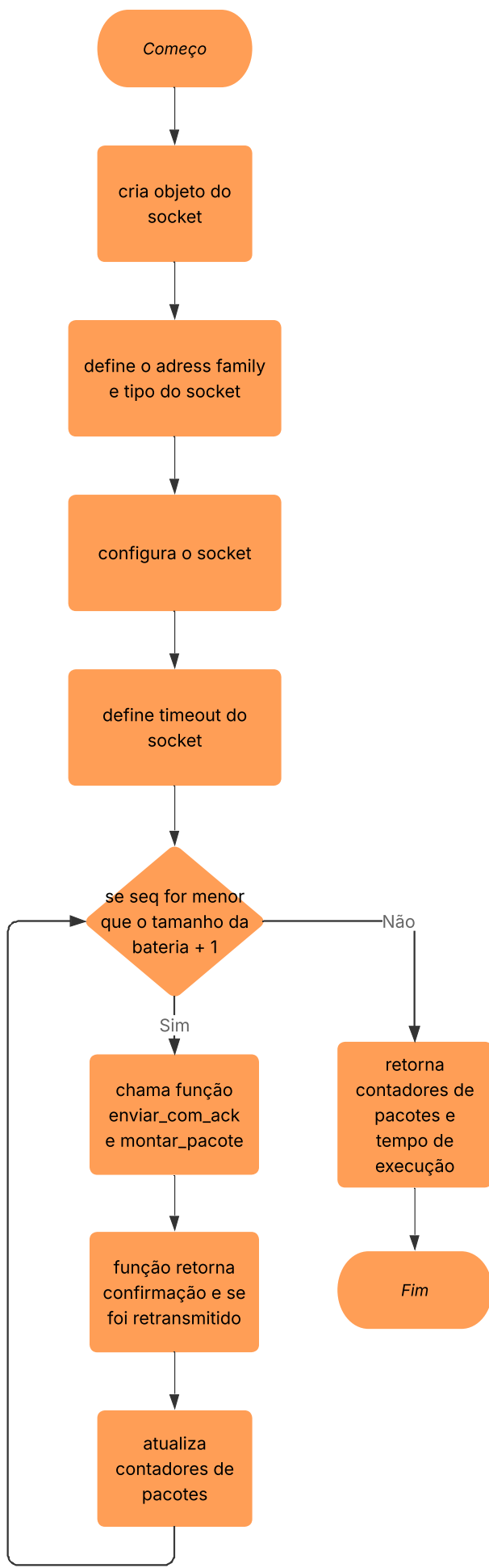
função rodar_udp
