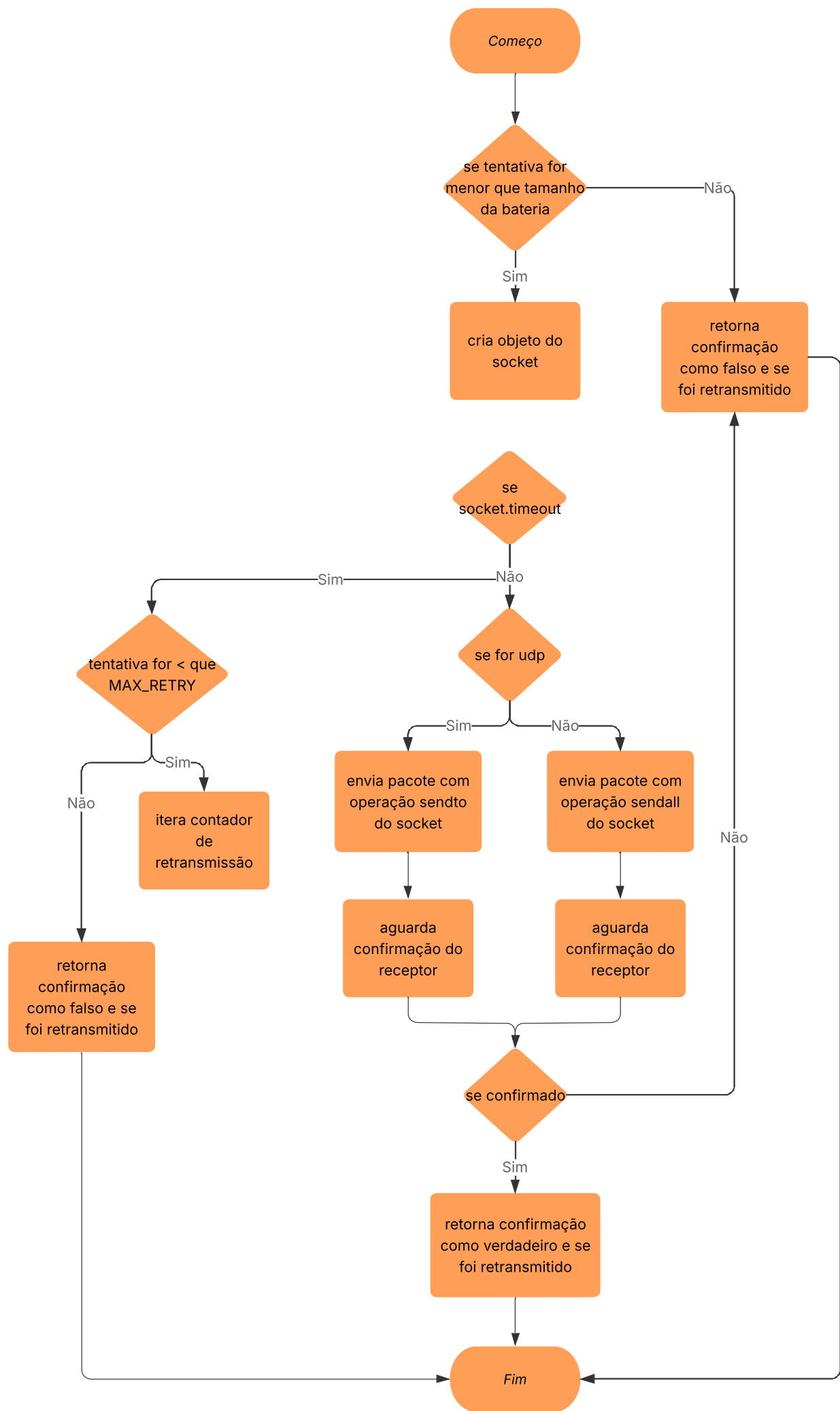
função enviar_com_ack
