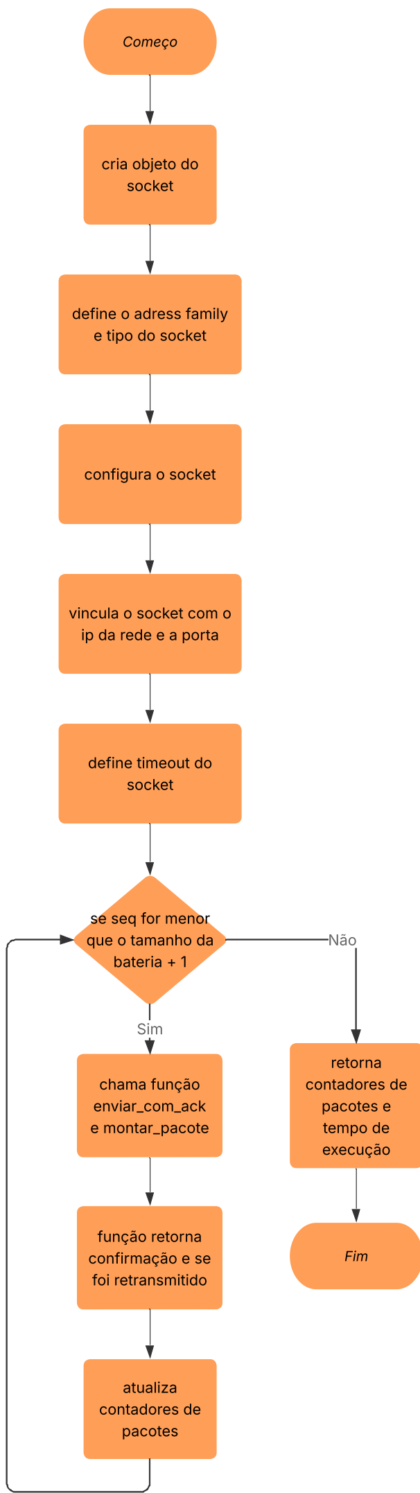
função rodar_tcp
