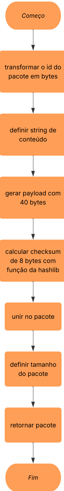
função montar_pacote
