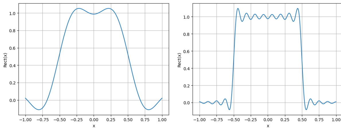
FIGURE 8 – TFI de \text{Rect}(x) avec bornes [-10, 10] (à gauche) et [-50, 50] (à droite)
