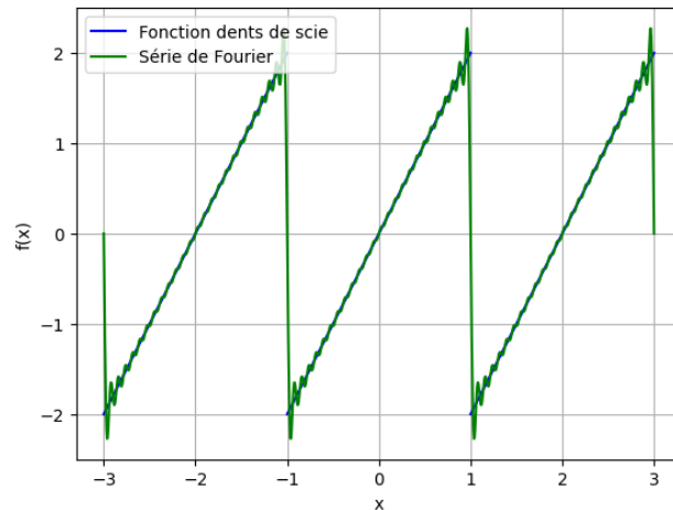
FIGURE 5 – Série de Fourier (25 premiers termes) de la fonction en dents de scie ( A = 2, T = 2 )
