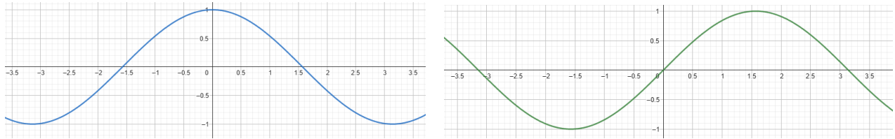
FIGURE 1 – \cos(x) (à gauche) et \sin(x) (à droite)
