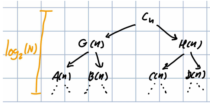
FIGURE 9 – Arbre de récursion de la FFT
