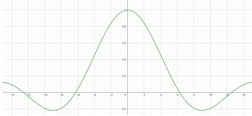
FIGURE 6 – c(\omega) pour le pulse rectangulaire ( \tau = 1 )
