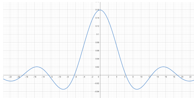
FIGURE 6 – c(\omega) pour le pulse rectangulaire ( \tau = 1 )
