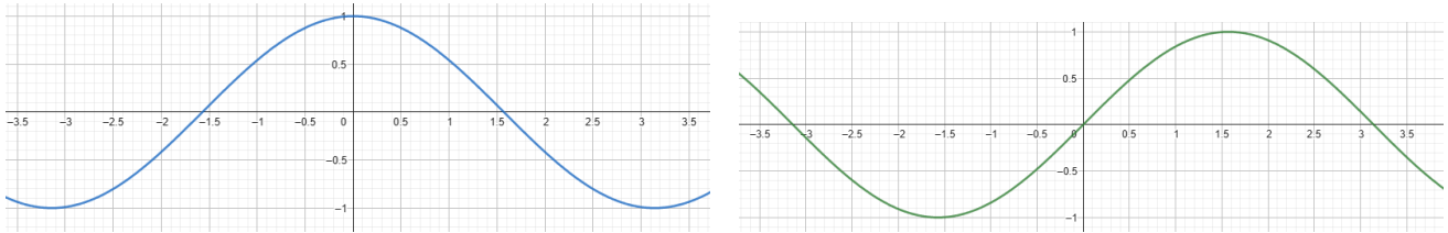
FIGURE 1 – La fonction \cos(x) (à gauche) et la fonction \sin(x) (à droite)
