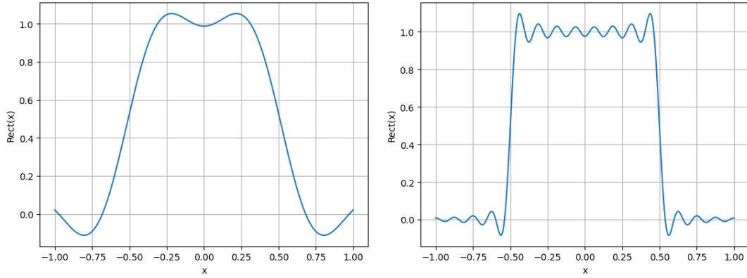
FIGURE 9 – TFI de \text{Rect}(x) ( \tau = 1 ) avec bornes [-10, 10] (à gauche) et [-50, 50] (à droite)
