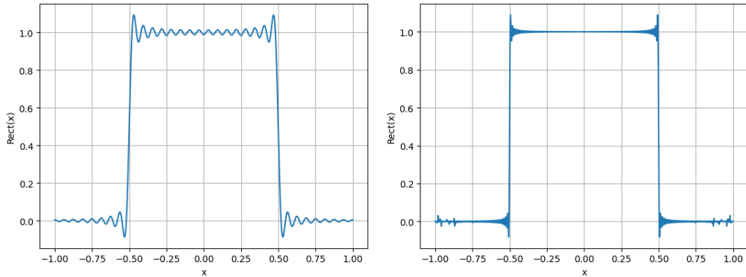
FIGURE 10 – TFI de \text{Rect}(x) ( \tau = 1 ) avec bornes [-100, 100] (à gauche) et [-500, 500] (à droite)
