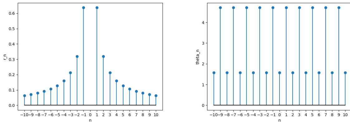
FIGURE 6 – Spectre de magnitude (à gauche) et de phase (à droite) des premiers c_n ( A = 2, T = 2 )
