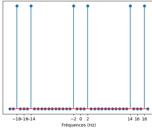
FIGURE 17 – Effet de l'échantillonnage sur le spectre de fréquence du signal de 2Hz
