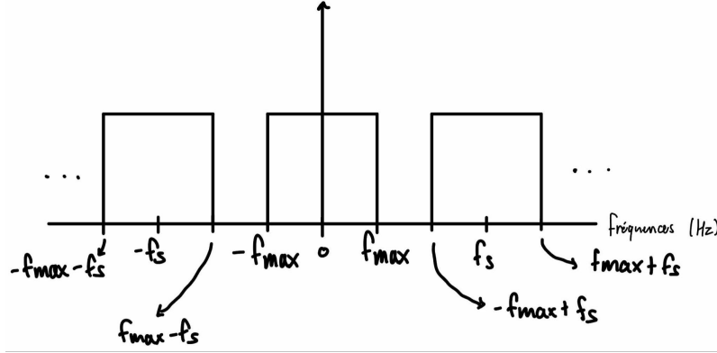
FIGURE 18 – Effet de l'échantillonnage sur le spectre de fréquence d'un signal quelconque avec une plage de fréquences limitée
