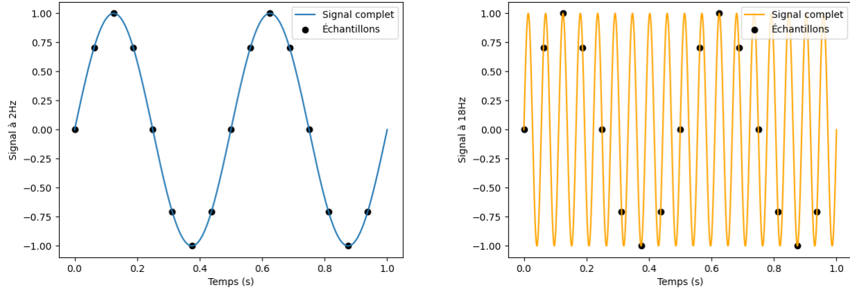
FIGURE 15 – Signal à 2Hz (à gauche) et signal à 18Hz (à droite) échantillonnés à f_s = 16\text{Hz} pour t \in [0, 1)
