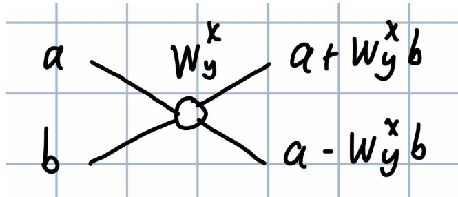
FIGURE 11 – Diagramme papillon général
