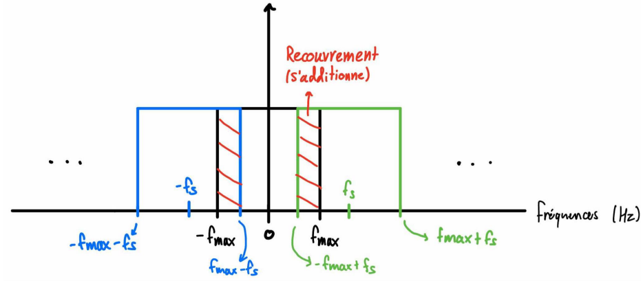
FIGURE 19 – Effet de l'échantillonnage sur le spectre de fréquence d'un signal quelconque avec une plage de fréquences limitée quand la fréquence d'échantillonnage n'est pas assez grande
