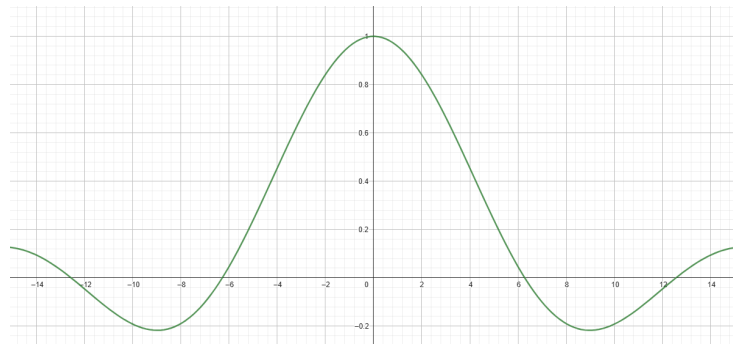
FIGURE 5 – c(\omega) pour le pulse rectangulaire ( \tau = 1 )
