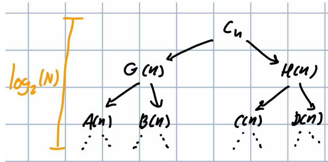
FIGURE 8 – Arbre de récursion de la FFT
