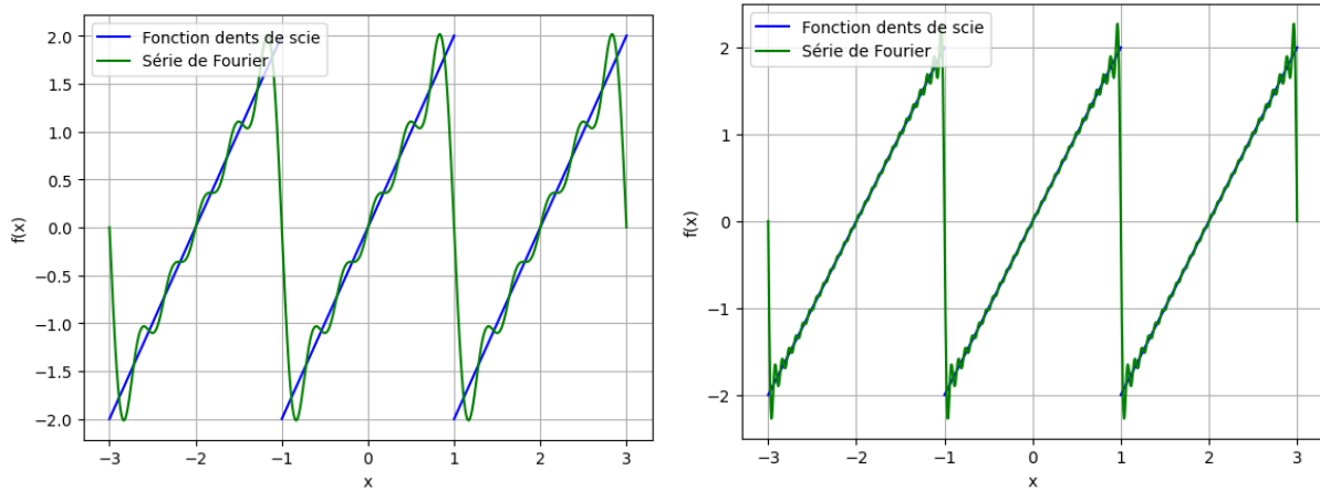
FIGURE 3 – Série de Fourier à 5 termes et à 25 termes de la fonction en dents de scie ( A = 2, T = 2 )
