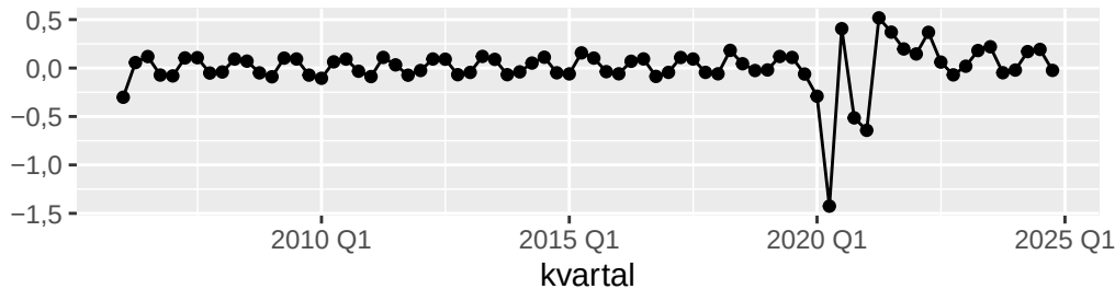
Residualer – Auto ARIMA – International (inkl. corona)
