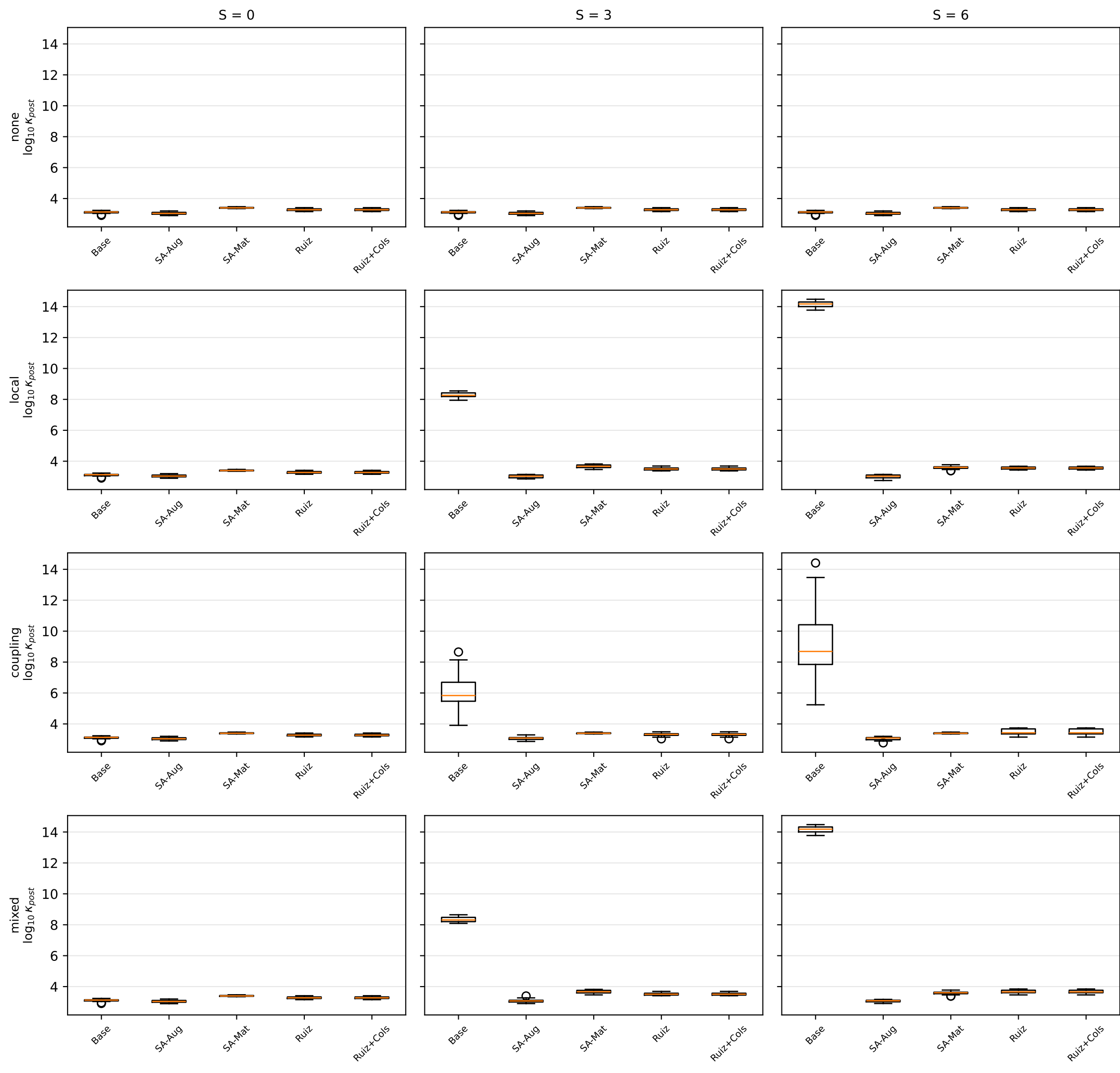
Condicionamiento posterior \log_{10} \kappa_{post} por variante (filas = pattern, columnas = S)
