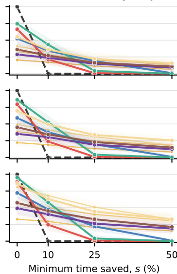
Classification (Gini)
