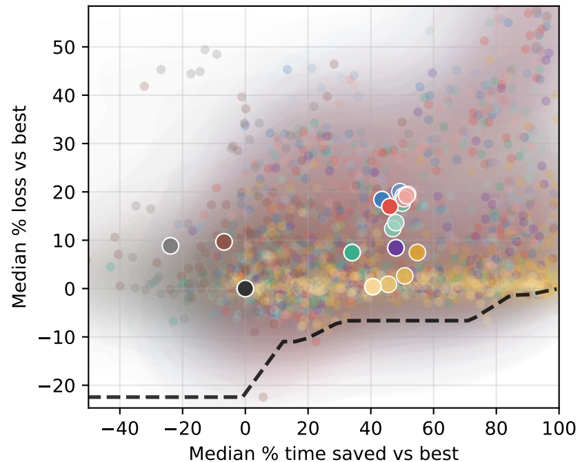
Gini
