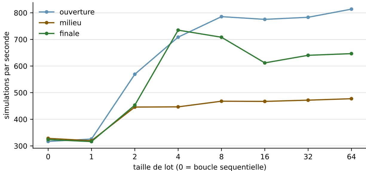
Balayage de la taille de lot, GPU, 400 simulations
