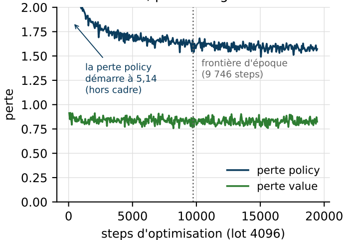
Pertes, prétraining Lichess
