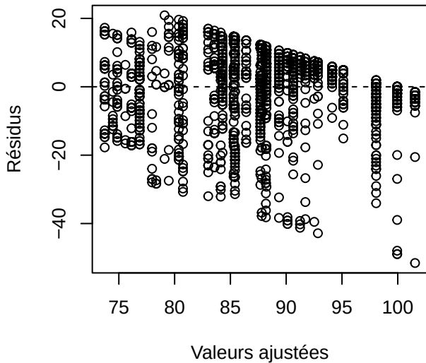
Résidus vs valeurs ajustées
