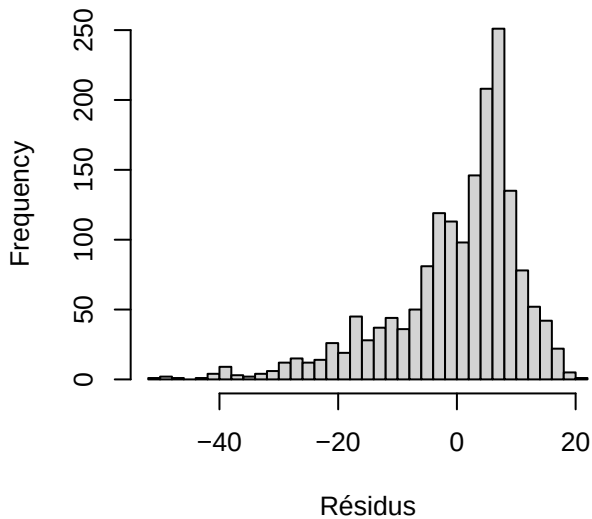
Distribution des résidus
