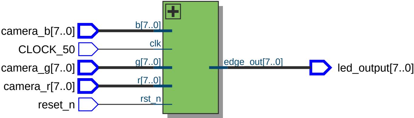
adas_pipeline_top:u_adas
