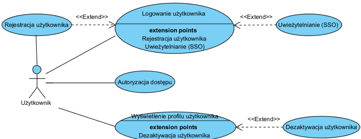
Rys. 5.3. Zarządzanie użytkownikami
