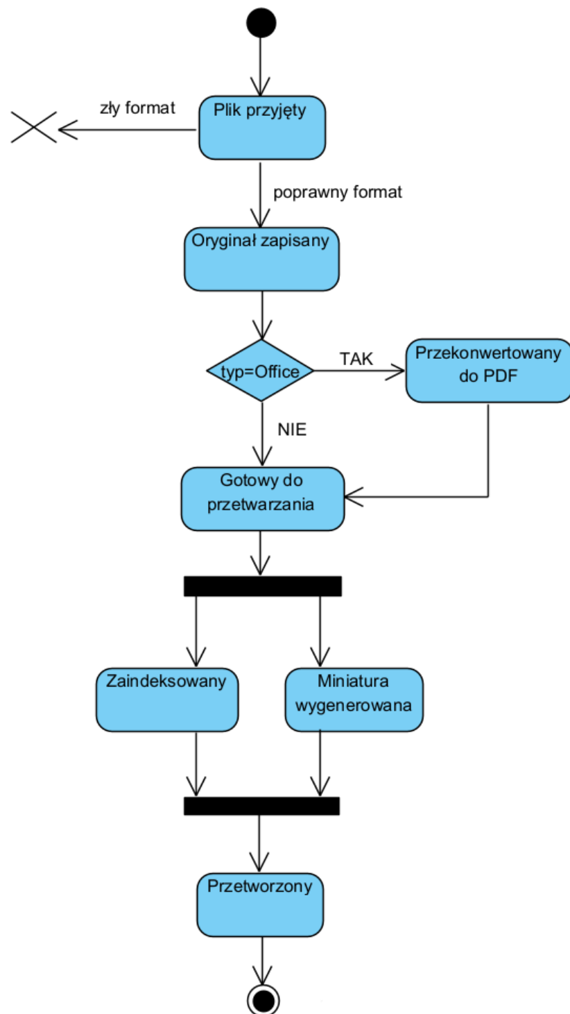
Rys. 5.15. Diagram stanów dokumentu
