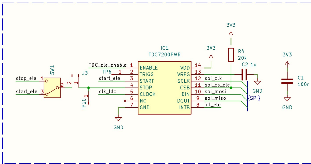
Abbildung 14: TDC Electrical Signal
