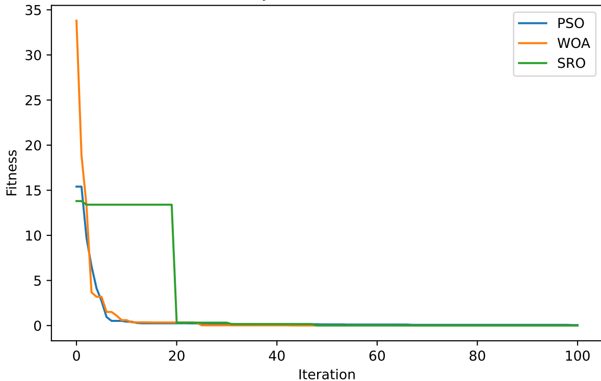
Best Fitness per MH F7 Mejor: SRO (0.00214)
