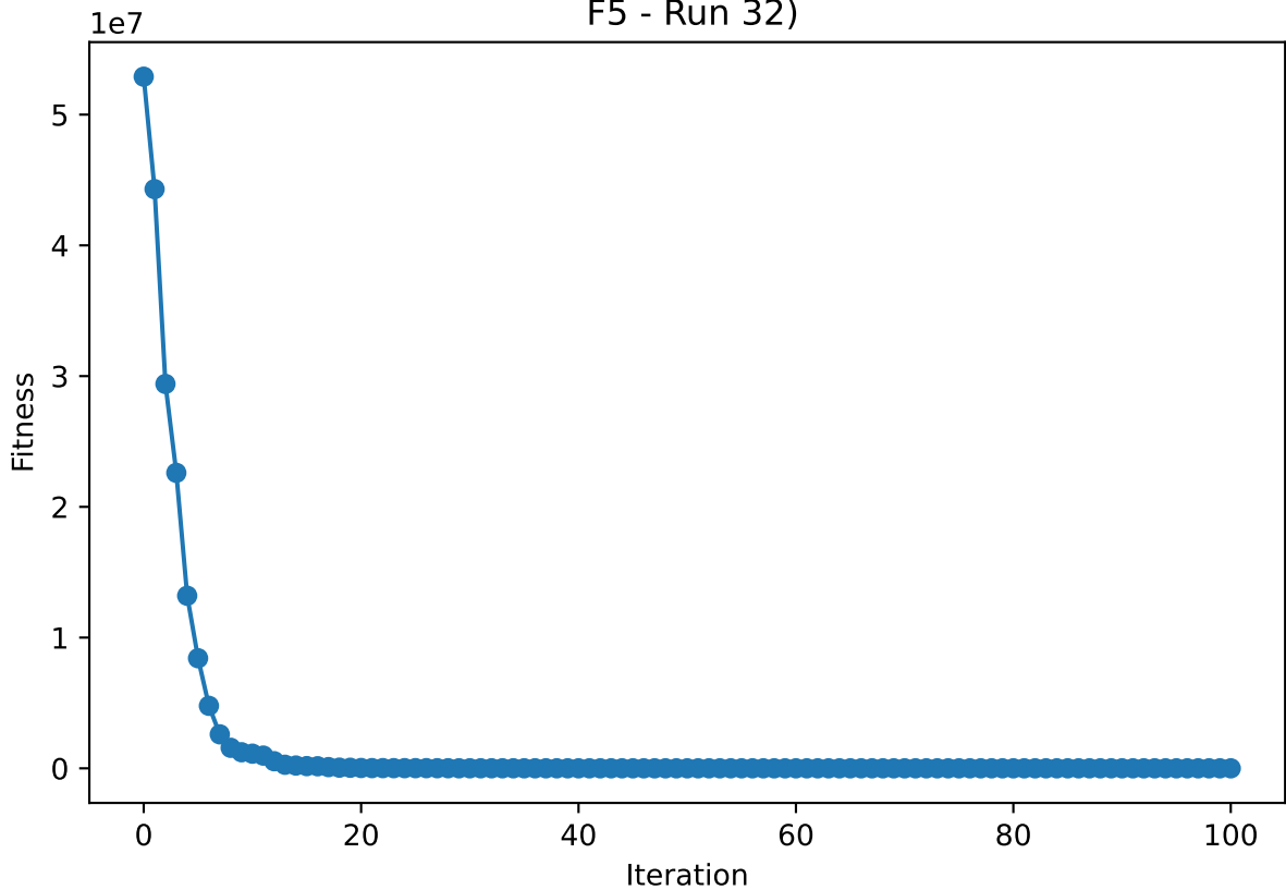
Convergence PSO F5 - Run 32)
