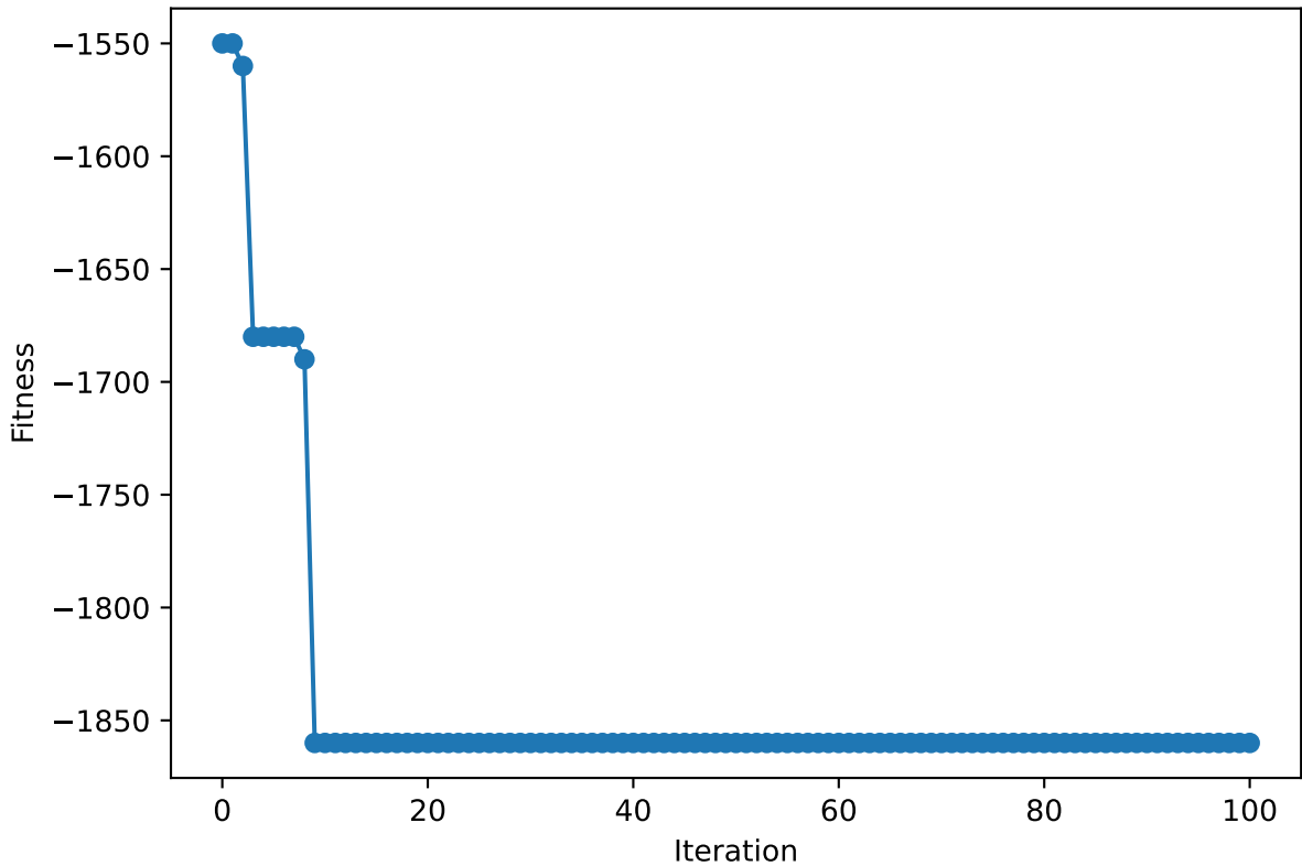
Convergence SRO F8 - Run 13)
