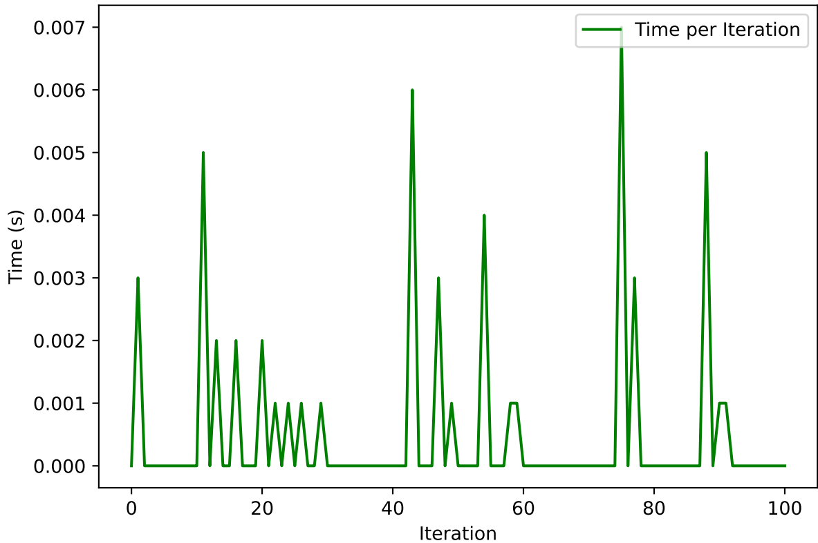
Time per Iteration PSO F1 - Run 30
