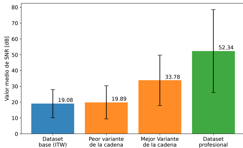
Figura 25. Comparación entre SNR de los datasets ITW y Profesional.
